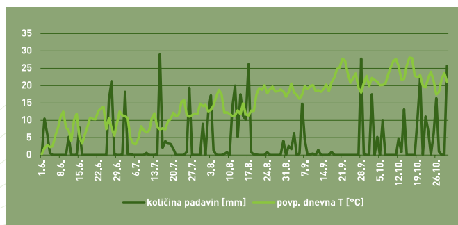
Slika 6: količina padavin v 24 urah (mm) in povprečna dnevna temperatura (°C) na vremenski postaji Novo mesto v vegetacijski sezoni 2023
