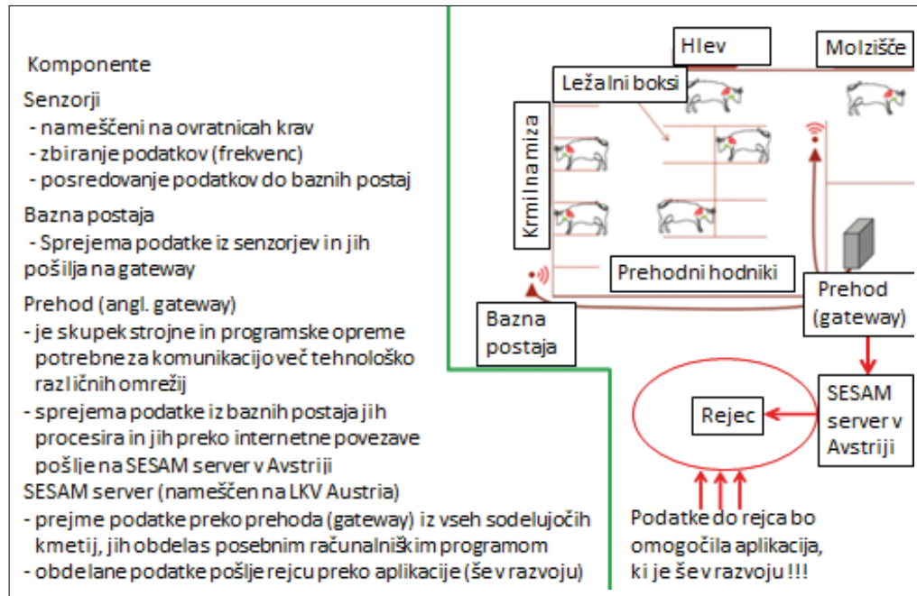
Shematski prikaz delovanja modularnih senzorskih sistemov, razvitih v okviru projekta SESAM
