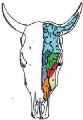
Votline v lobanji krave: obnosna, čeljustna, nebna, solzna, zgornja nosna, čelna, sinusna in votline v rogovih.
